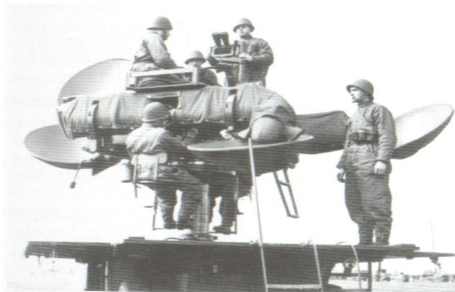
Rys. 4. Nasłuchownik przeciwlotniczy
